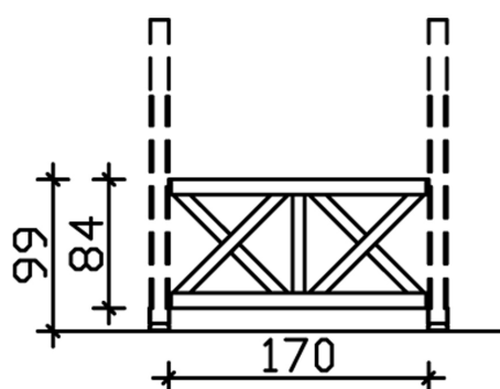
Bemassung
