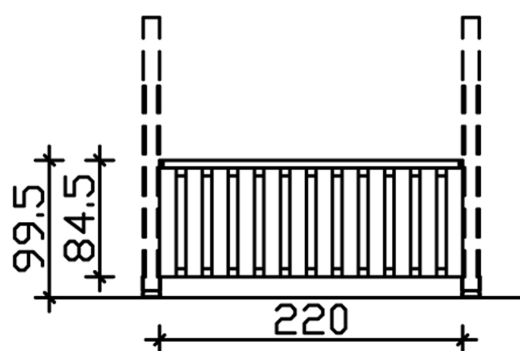
Bemassung
