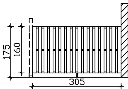
Bemassung
