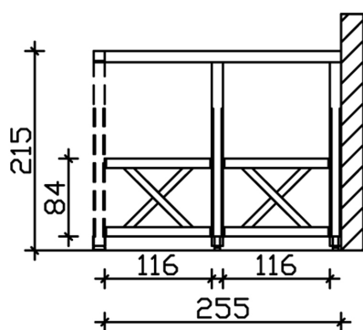
Bemassung
