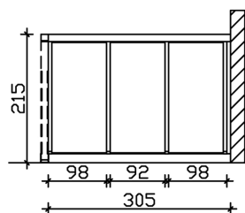
Bemassung
