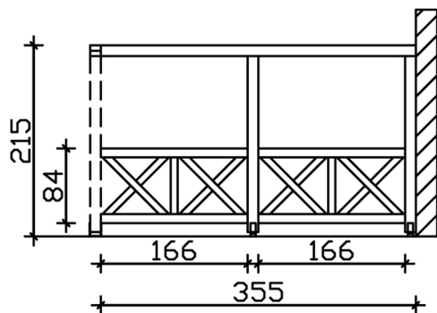
Bemassung
