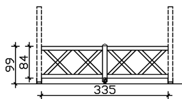
Bemassung
