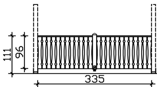
Bemassung
