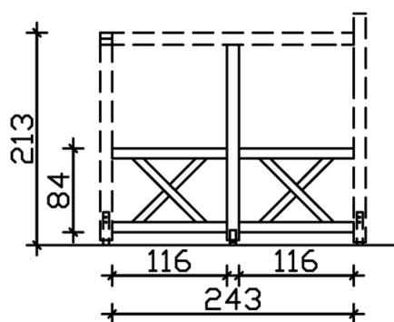
Bemassung
