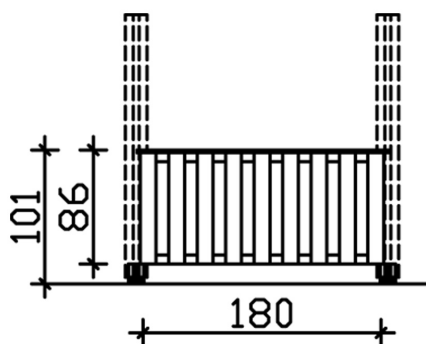
Bemassung
