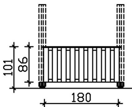
Bemassung
