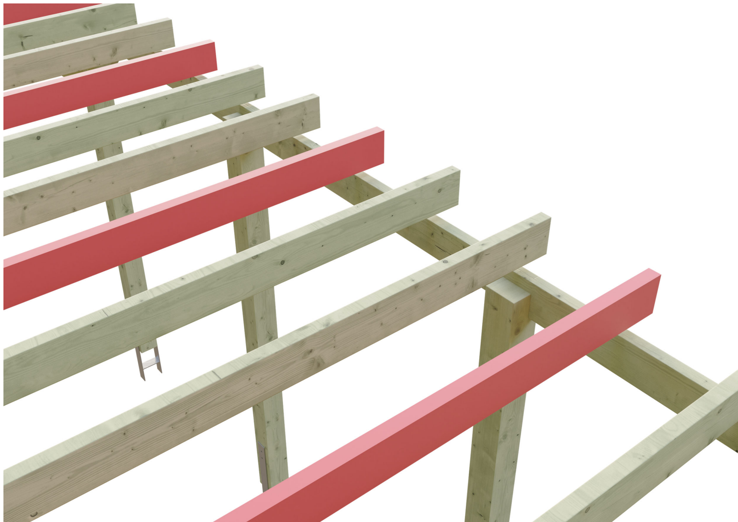
Schneelasterhöhung
