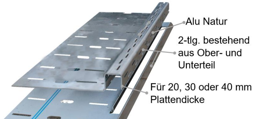
Abbildung 1: Stufenprofil Ober- und Unterteil
