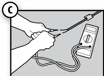
Widerstand mittels eines Ohmmeters messen
