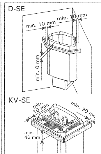
Figure 6. Safety railing Abbildung 6. Schutzgeländer
