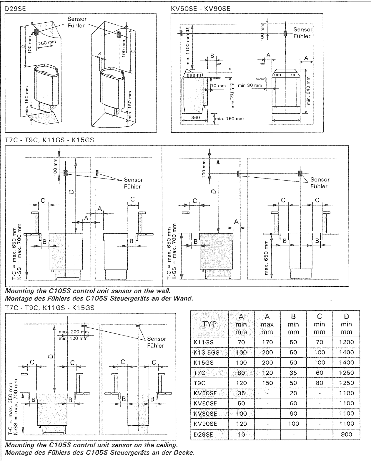
Figure 4. Safety distances from the heater Abbildung 4. Sicherheitsmindestabstände des Saunaofens
